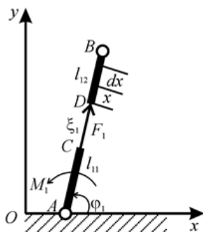
Рисунок 1. Модель звена сноубордиста переменной длины на плоскости
