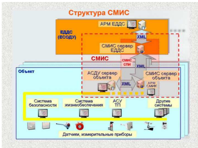
Рисунок 1. Укрупненная структура системы мониторинга инженерных систем (СМИС) уникальных зданий и сооружений (Коргин А.В., 2011 [6])
